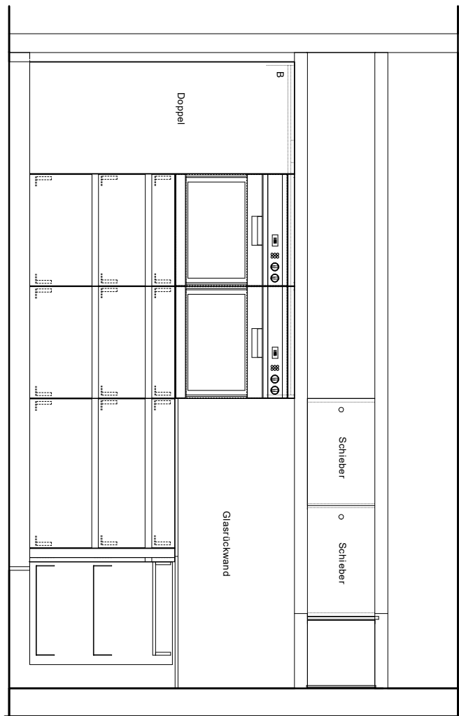
Ansicht A
