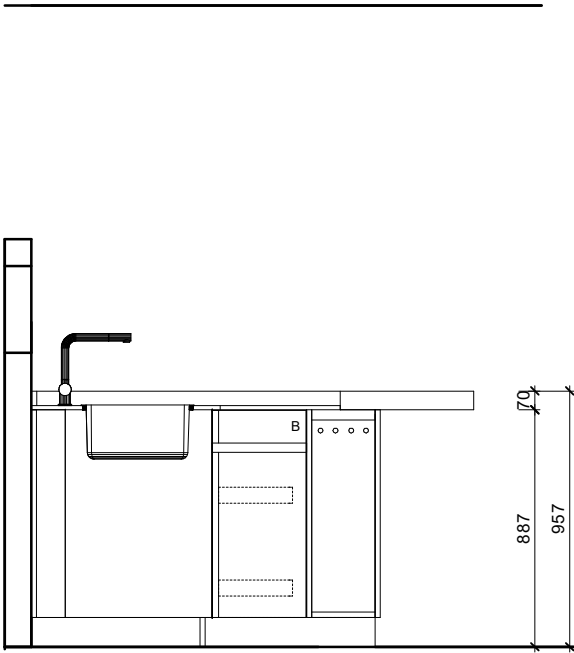
Ansicht D
