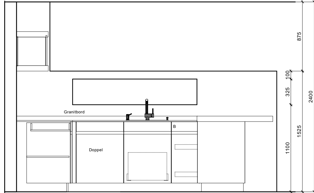
Ansicht C
